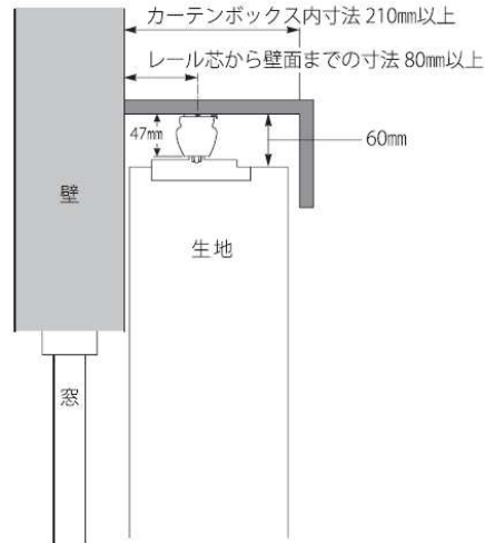
カーテンボックスの内寸法が210mm以上の場合
