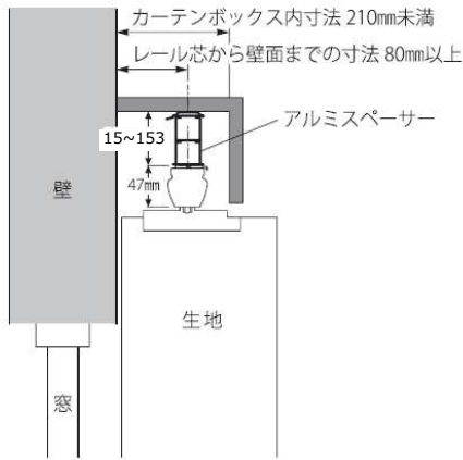
カーテンボックスの内寸法が210mm未満の場合
