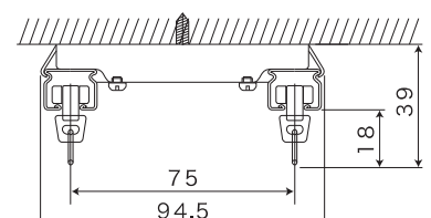
天井付ダブルブラケット75
