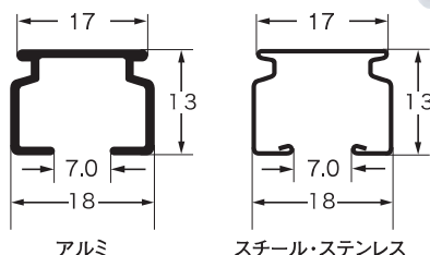
レール断面図(単位:mm)
