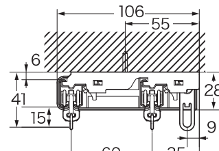
サイドユニットW 天井付Fダブルブラケット
