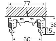
天井付ダブルブラケット
