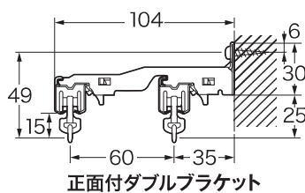
正面付ダブルブラケット
