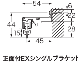
正面付EXシングルブラケット
