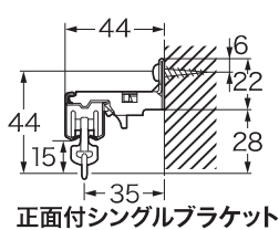
正面付シングルブラケット
