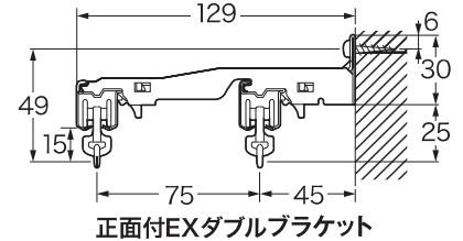
正面付EXダブルブラケット
