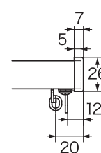
サイドユニットW
