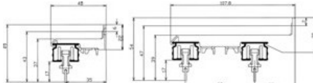
正面付シングルブラケット 正面付ダブルブラケット
