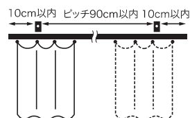
ブラケット取付け間隔と カーテン許容荷重
