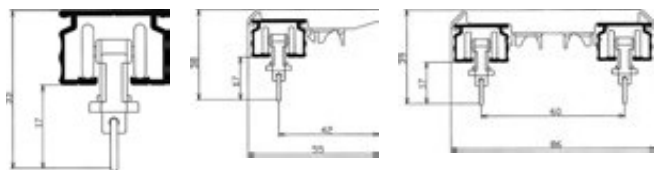
天井直付 天井付シングルブラケット 天井付ダブルブラケット
