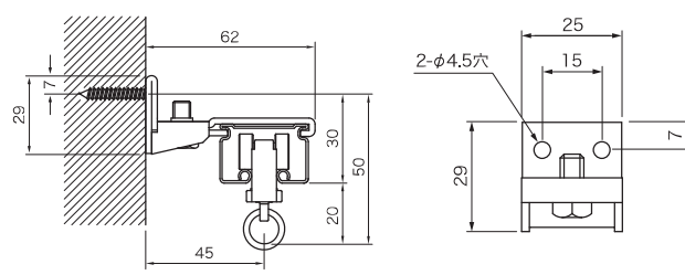
シングルブラケット付 (ブラケット幅=25mm)
