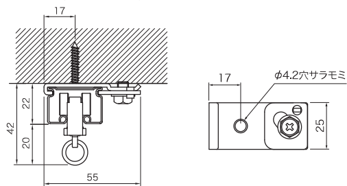
天井ブラケット付 (ブラケット幅=25mm)
