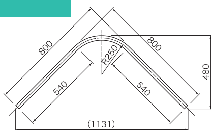
カーブレール
