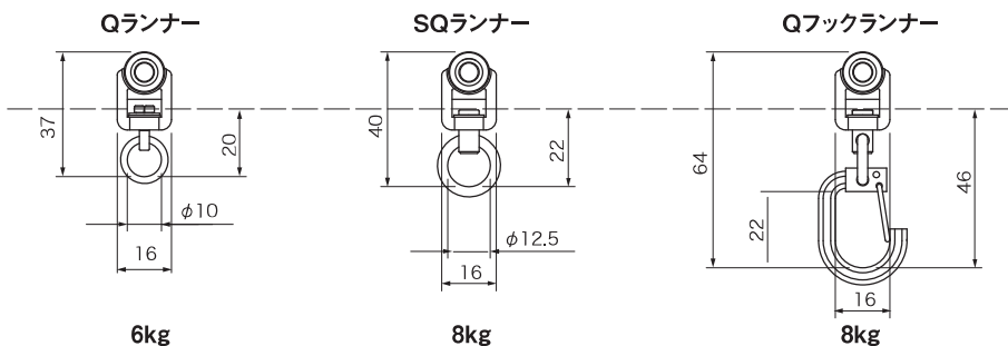
ランナー1個当りの許容荷重
