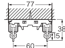
天井付ダブルブラケット
