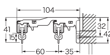
正面付EXシングルブラケット
