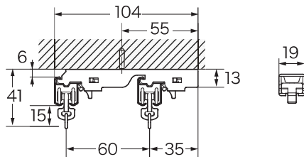
天井付Fダブルブラケット
