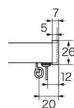
サイドユニットW
