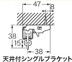
天井付シングルブラケット
